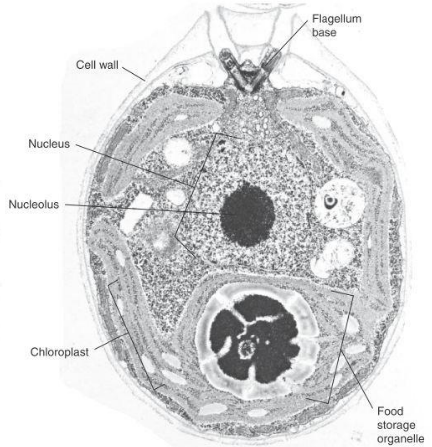
Chlamydomonas
